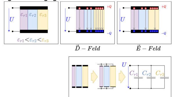
Fig. 23: längsgeschichteter Kondensator
