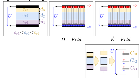
Fig. 22: quergeschichteter Kondensator
