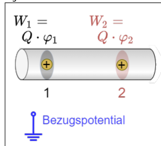
Fig. 9: elektrisches Potential
