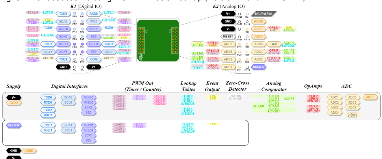
Fig. 3: Interfacebeschreibung MCB 1x1 Basis Hookup (Version 1.0 für AVR32DB)
