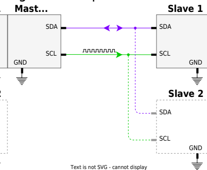
Fig. 3: Konzeptbild I2C
