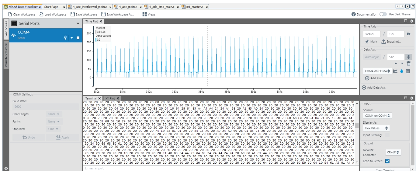
Fig. 31: Data Visualizer
